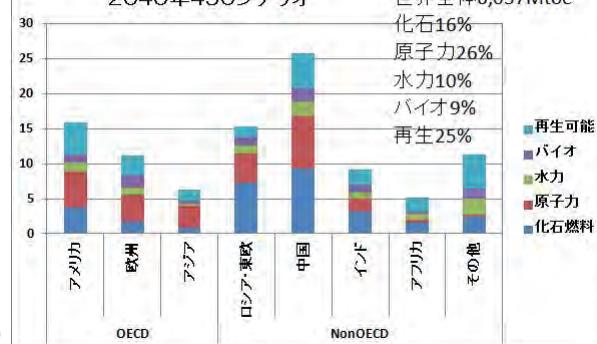
世界全体の発電量に対する割合(%) 2040年450シナリオ
